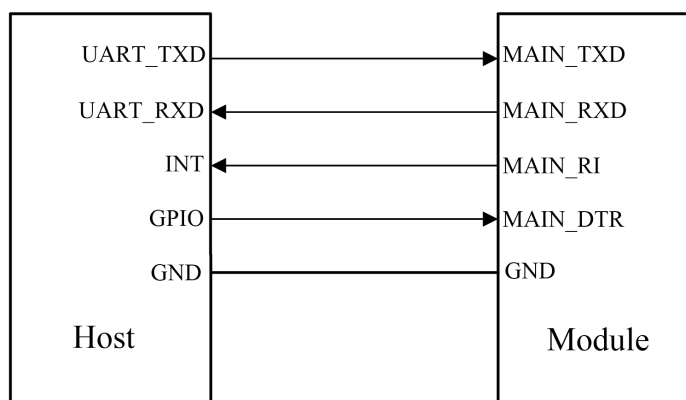
图 3-15A UART 接口休眠唤醒硬件连接图
