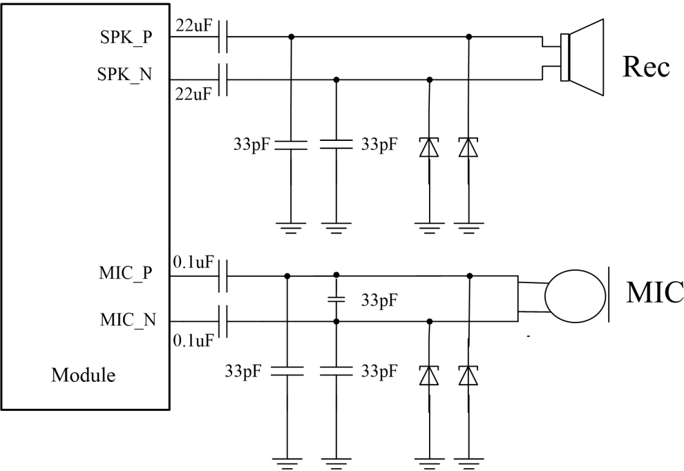
图 3-20 模拟语音电路图
