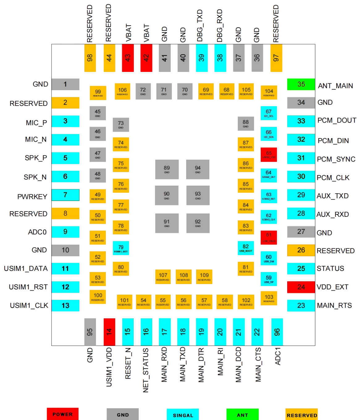
图 3-1 CLM920_LV9 模块管脚分布图（TOP 透视）
