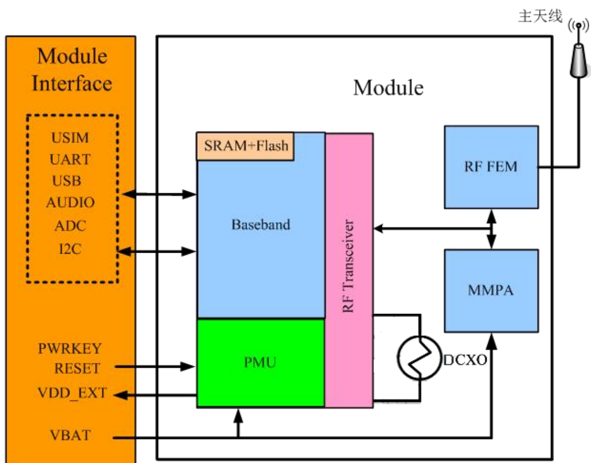
图 2-1 CLM920_LV9 模块功能框图
