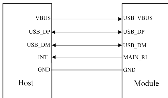
图 3-15C 支持 MAIN_RI 唤醒功能硬件连接图
