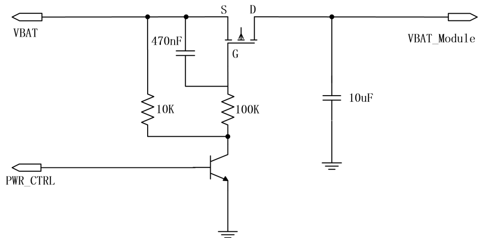
图 3-5 PMOS 管控制电源开关参考电路
