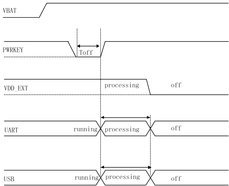
图 3-11 关机时序图
