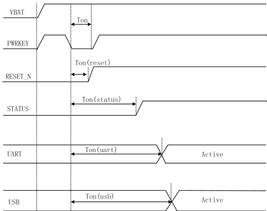
图 3-8 开机时序图
