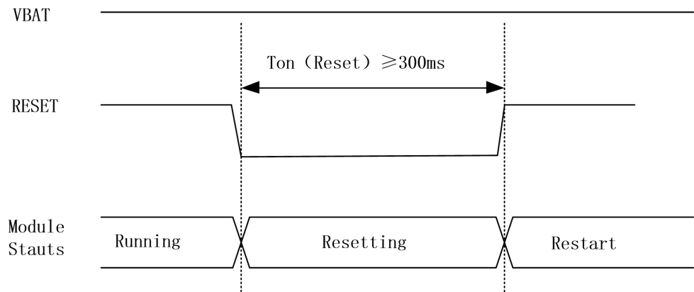
图 3-7 复位时序图
