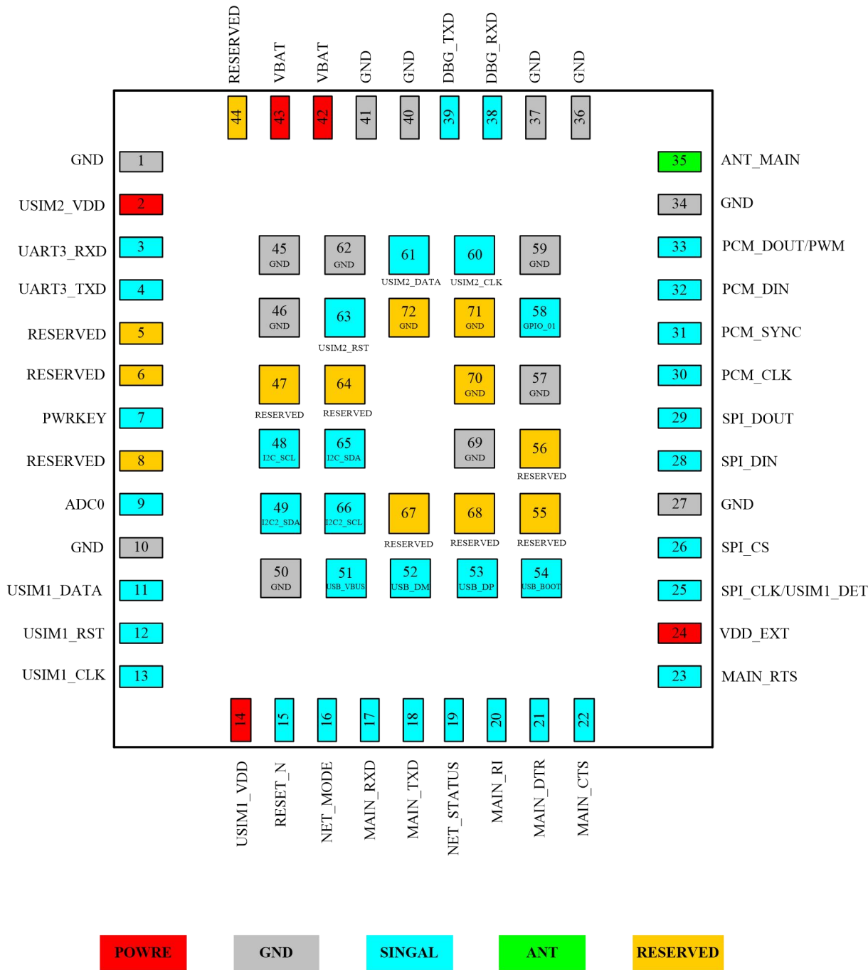
图 3-1 CLM920_HV9 V2 模块管脚分布图（TOP 透视）
