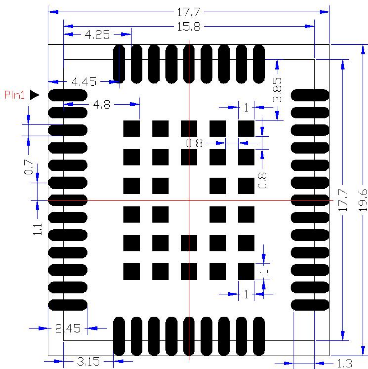
图 6-4 模块推荐封装(单位: 毫米)
