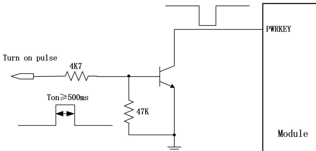
图 3-9 开集驱动开机参考电路
