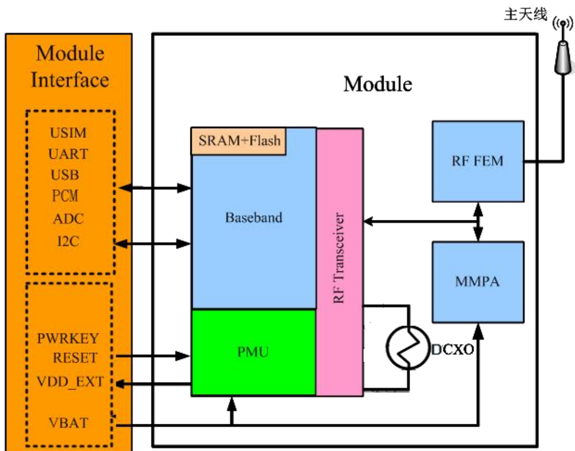
图 2-1 CLM920_HV9 V2 模块功能框图
