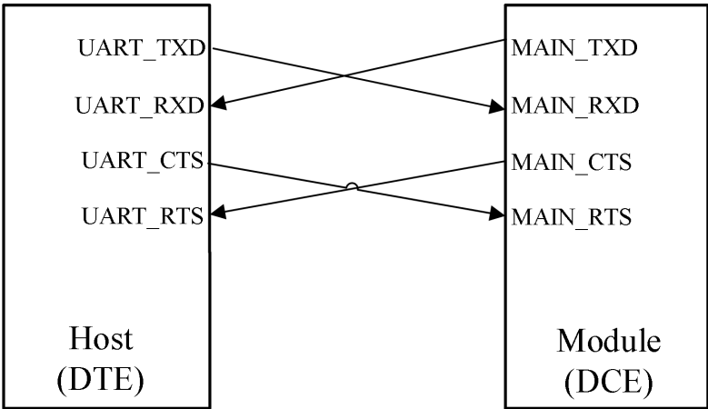
图 3-13 串口设计图
