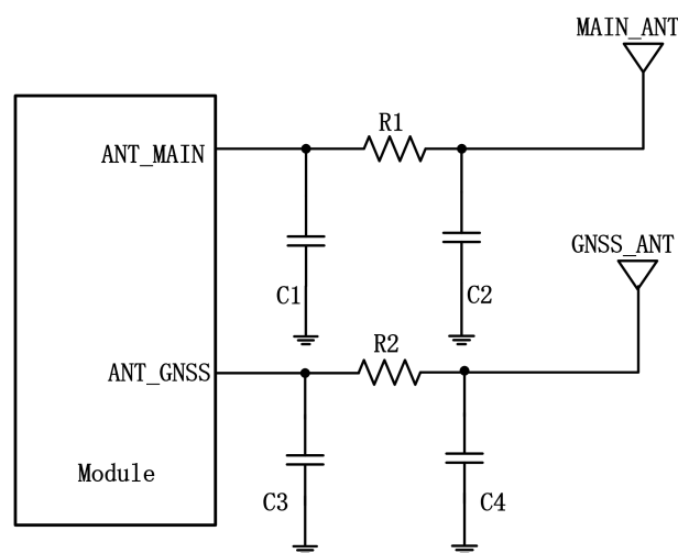
图 3-22 天线匹配电路
