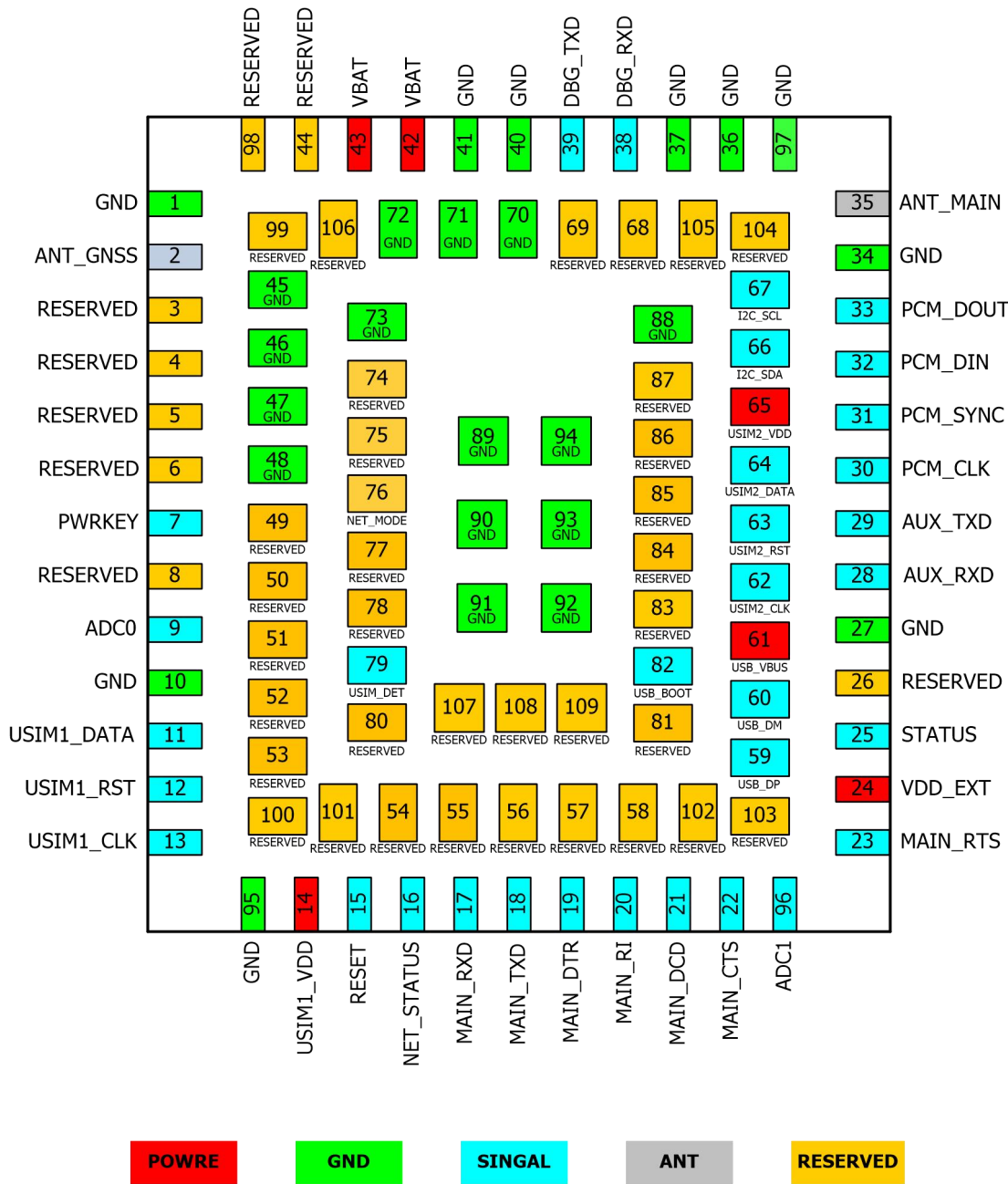
图 3-1 CLM920 HV9 G 模块管脚分布图（TOP 透视）
