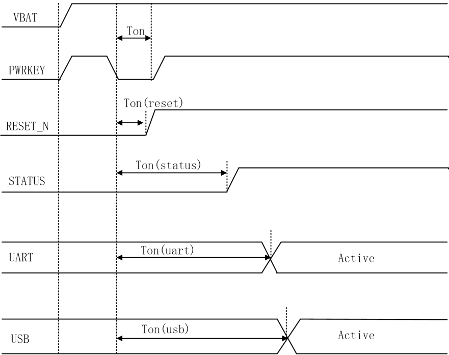
图 3-8 开机时序图
