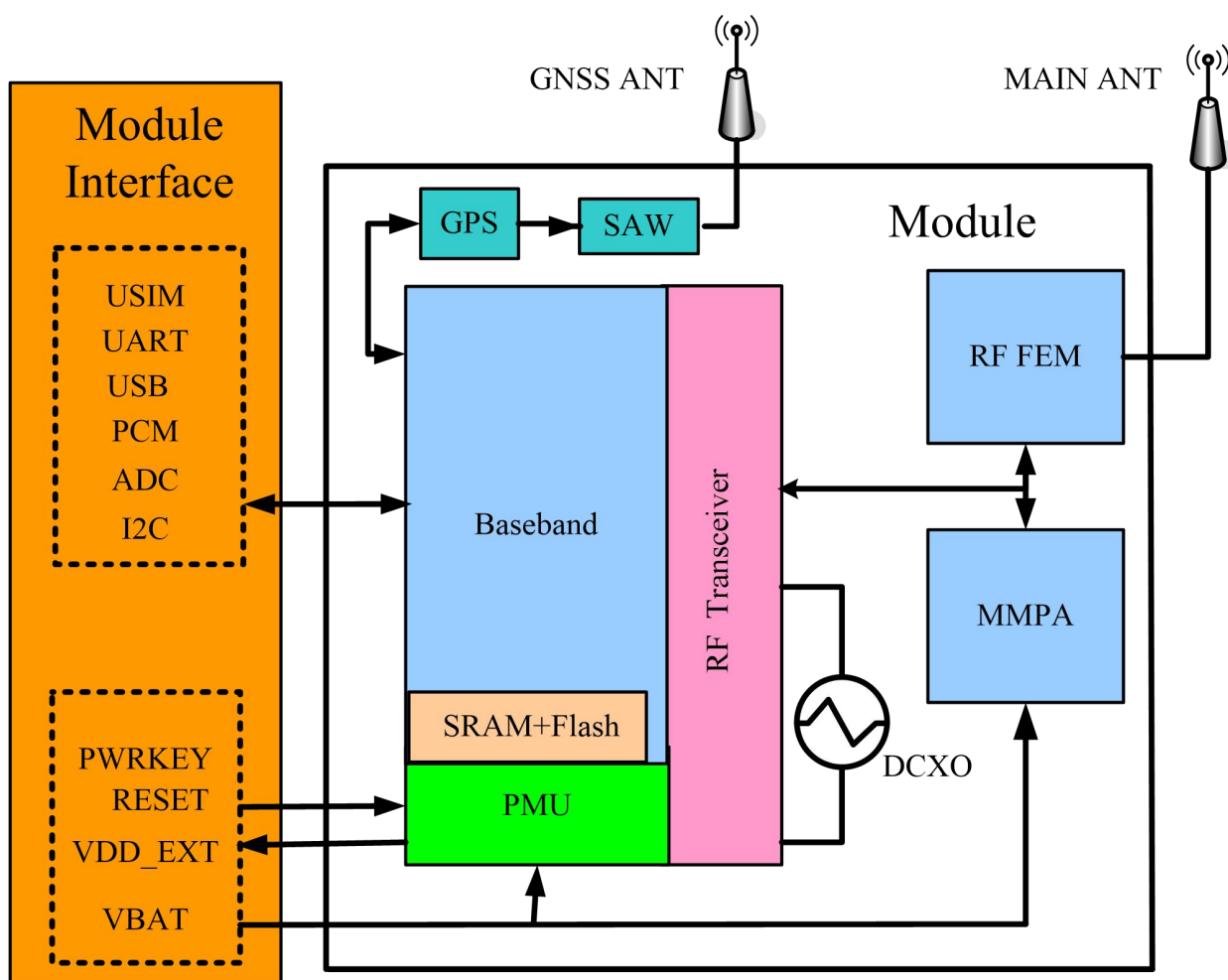
图 2-1 CLM920 HV9 G 模块功能框图
