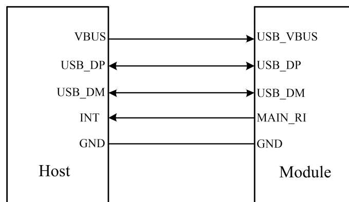
图 3-15C 支持 MAIN_RI 唤醒功能硬件连接图
