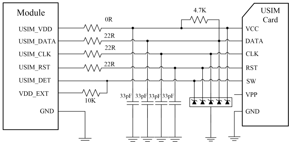
图 3-16 USIM 设计电路图
