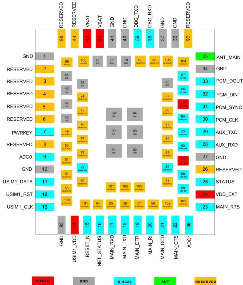
图 3-1 CLM920_HV9 模块管脚分布图（TOP 透视）
